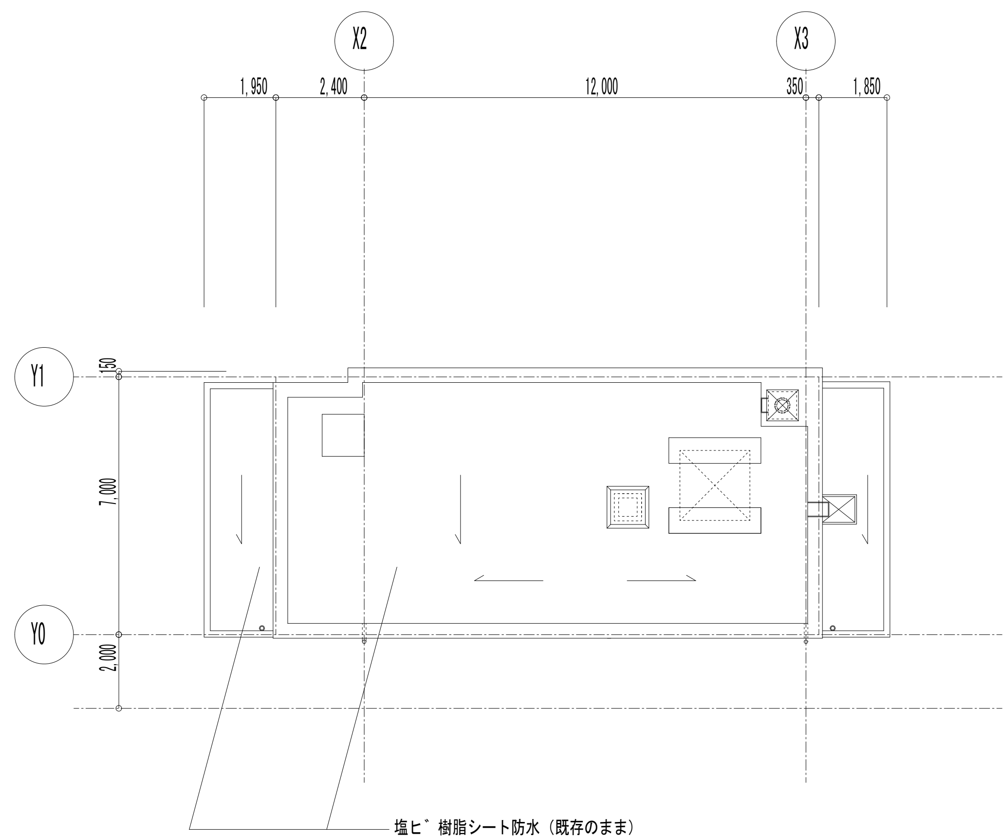
改修後 屋根伏図
