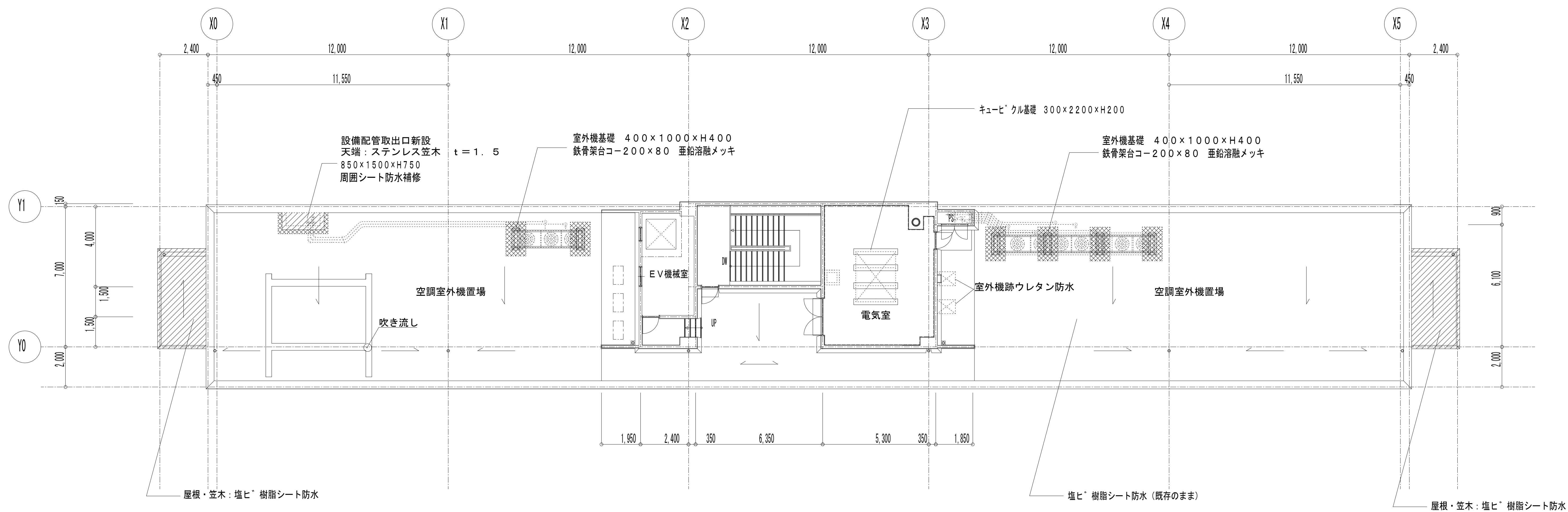
改修後 R F 平面図
