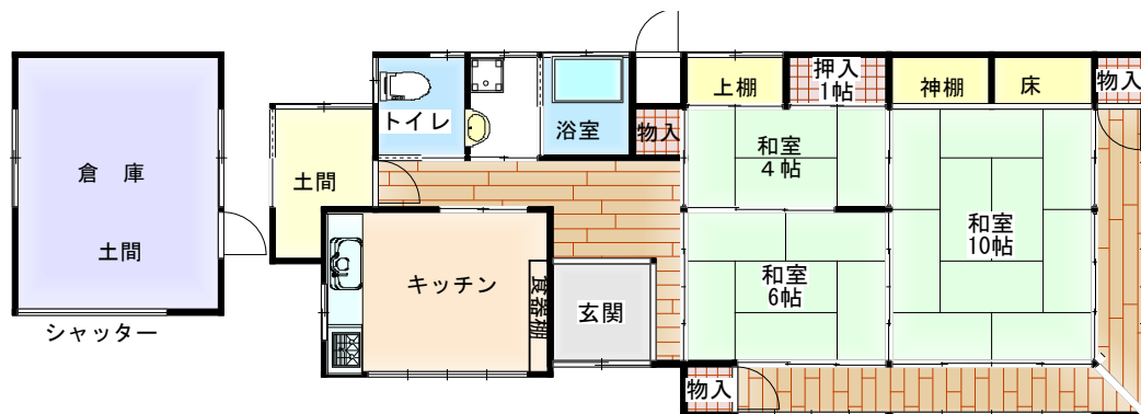
間取り図
