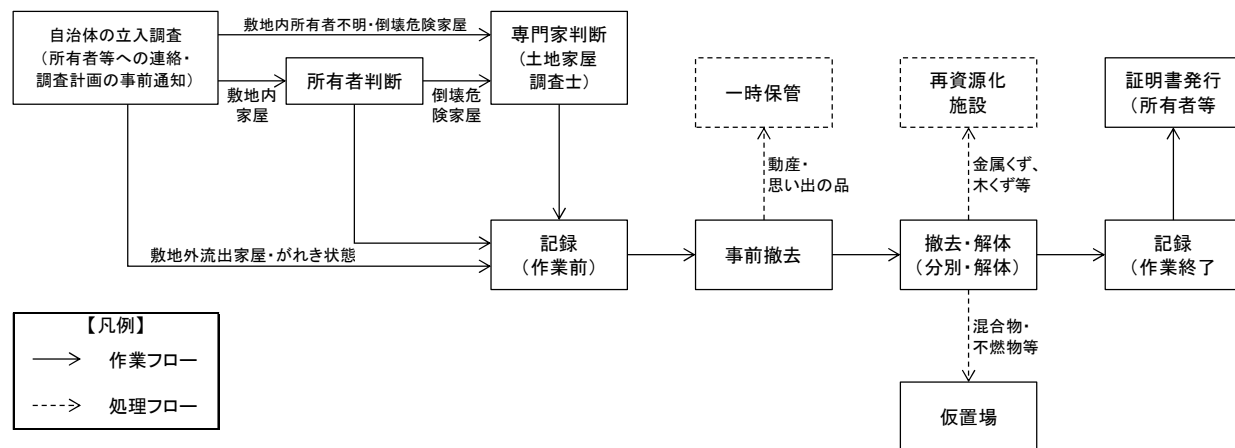
図 2.6.3 倒壊家屋等の解体作業フロー
