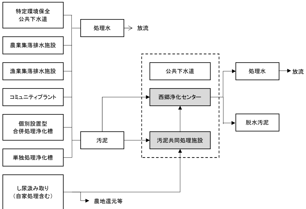
図 1.3.2 本町の生活排水処理フロー（令和3年度以降）
