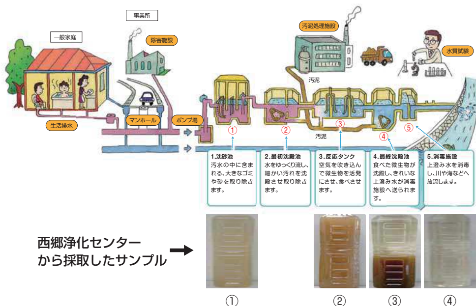
図1：排水の浄化過程
