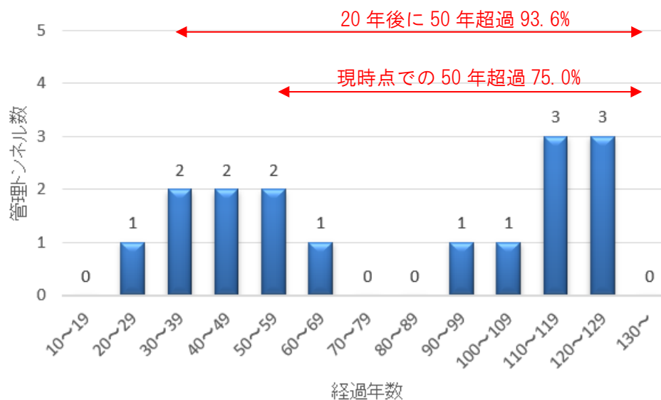
図 2-2 経過年数別のトンネル本数分布
